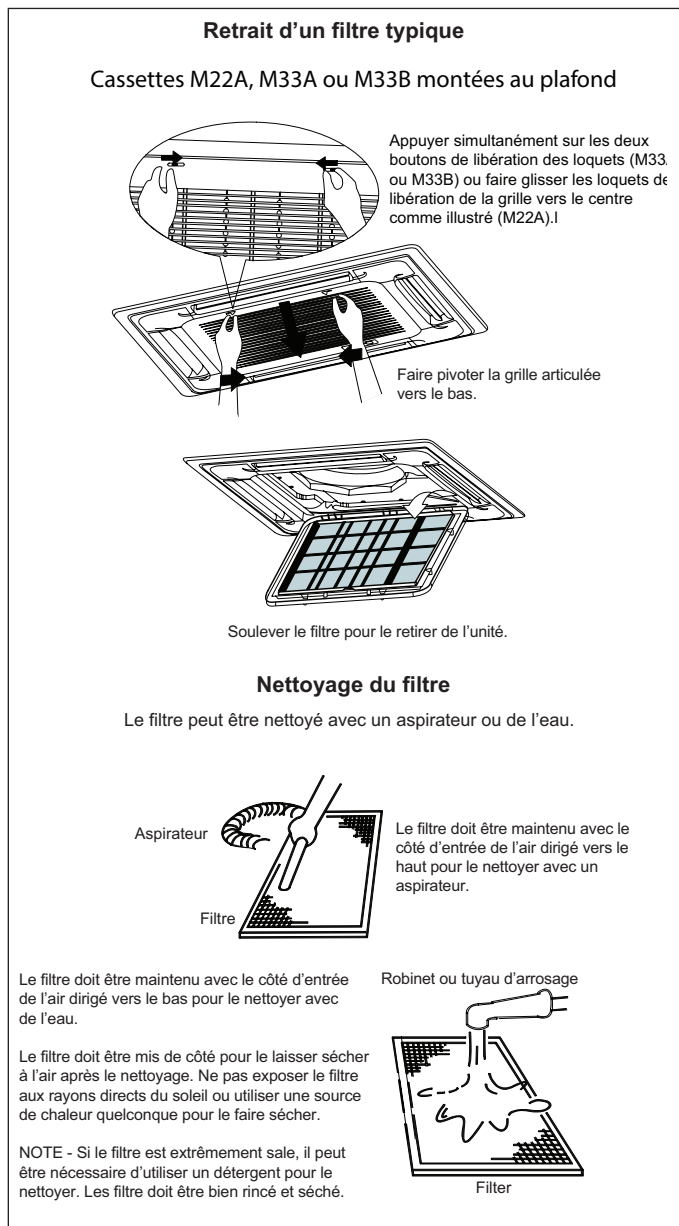
Figure 5. Retrait et nettoyage d'un filtre typique
