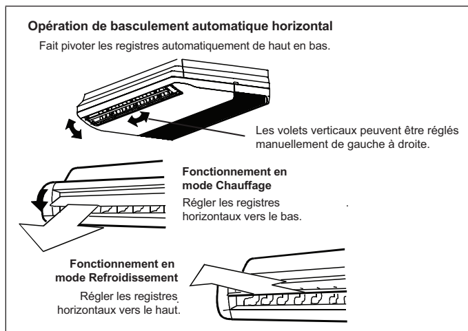
Figure 3. Unités de sol ou de plafond
